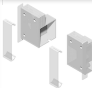
Wieszak osłony i żaluzji drewnianej Bracketforcoverandwooden blinds Монтажное крепление для планки и деревянные жалюзи
